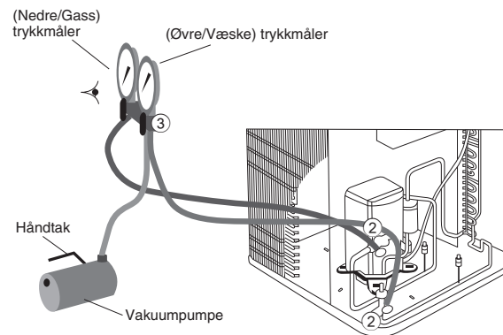
Eksempel på innstilling for deteksjon av kjølemediumlekkasje.
